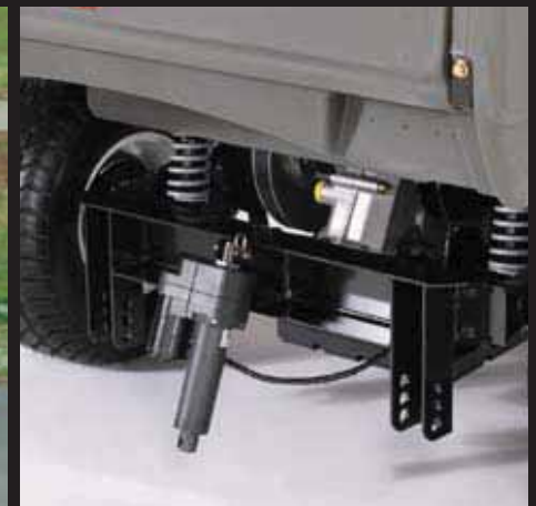
後部リフト
